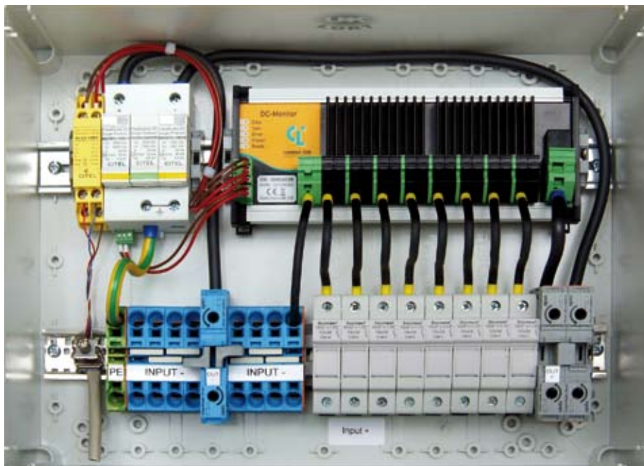
Keine aufwendige Montage mehr: Der „DC-Monitor“ passt auch in kleinere Schaltschränke.
